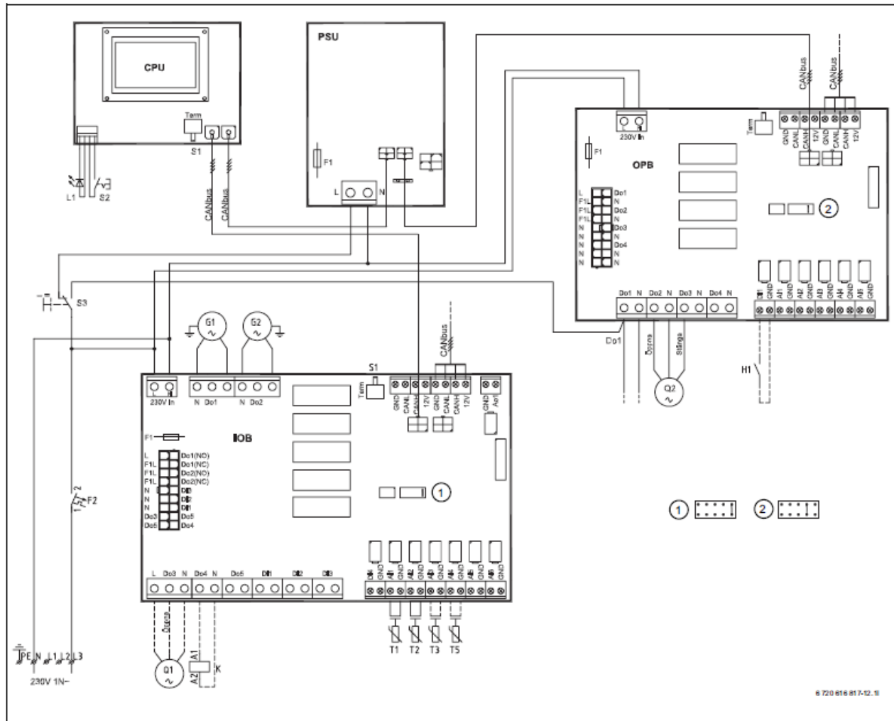
Bild 61 Kretsschema styrschåp, shuntat tillskott
