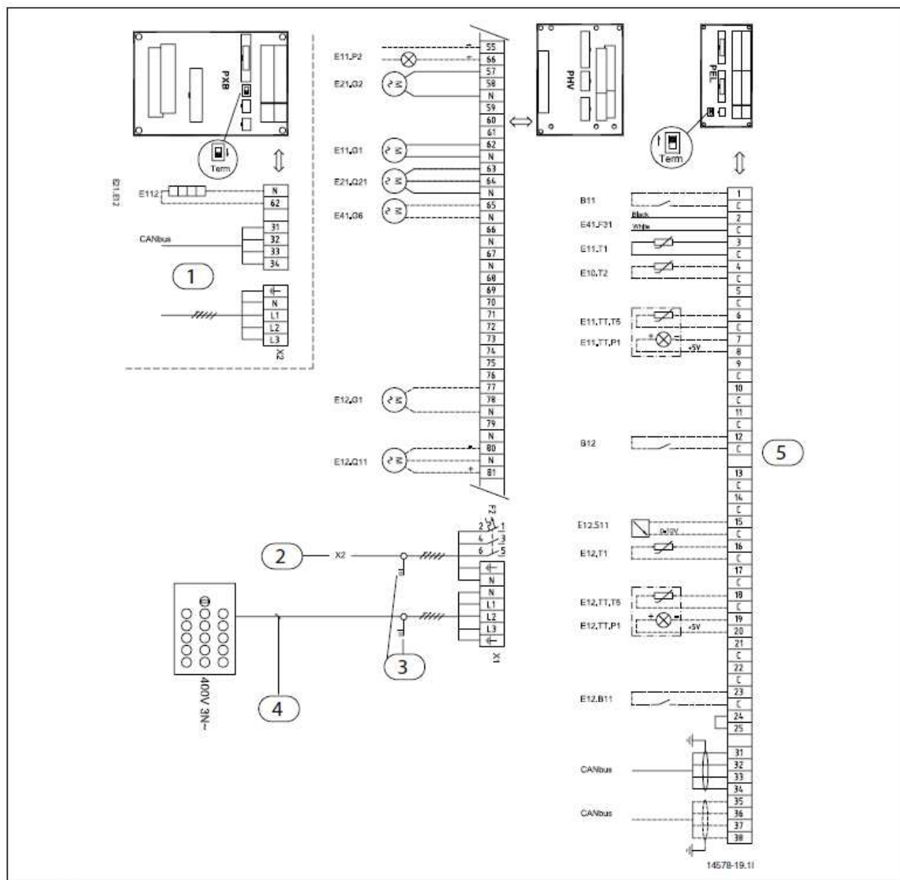
Bild 39 Externa anslutningar
