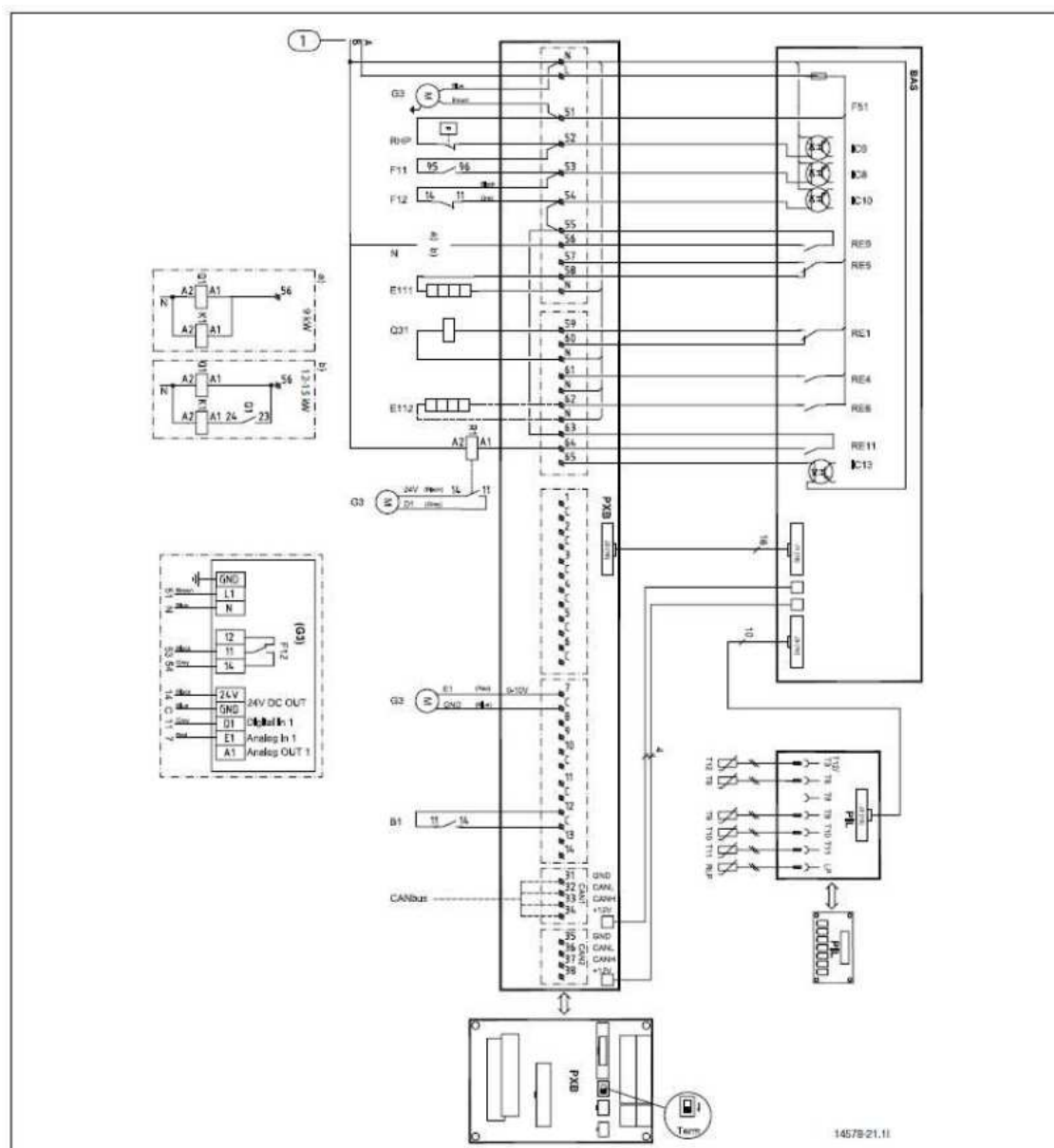
Bild 35 Anslutningar värmepump
