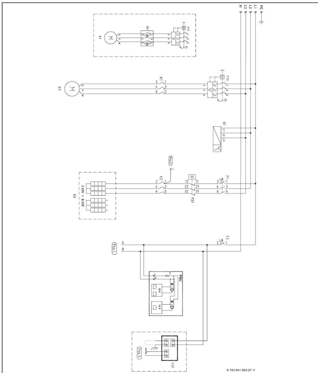
Bild 45 Internt elschema
