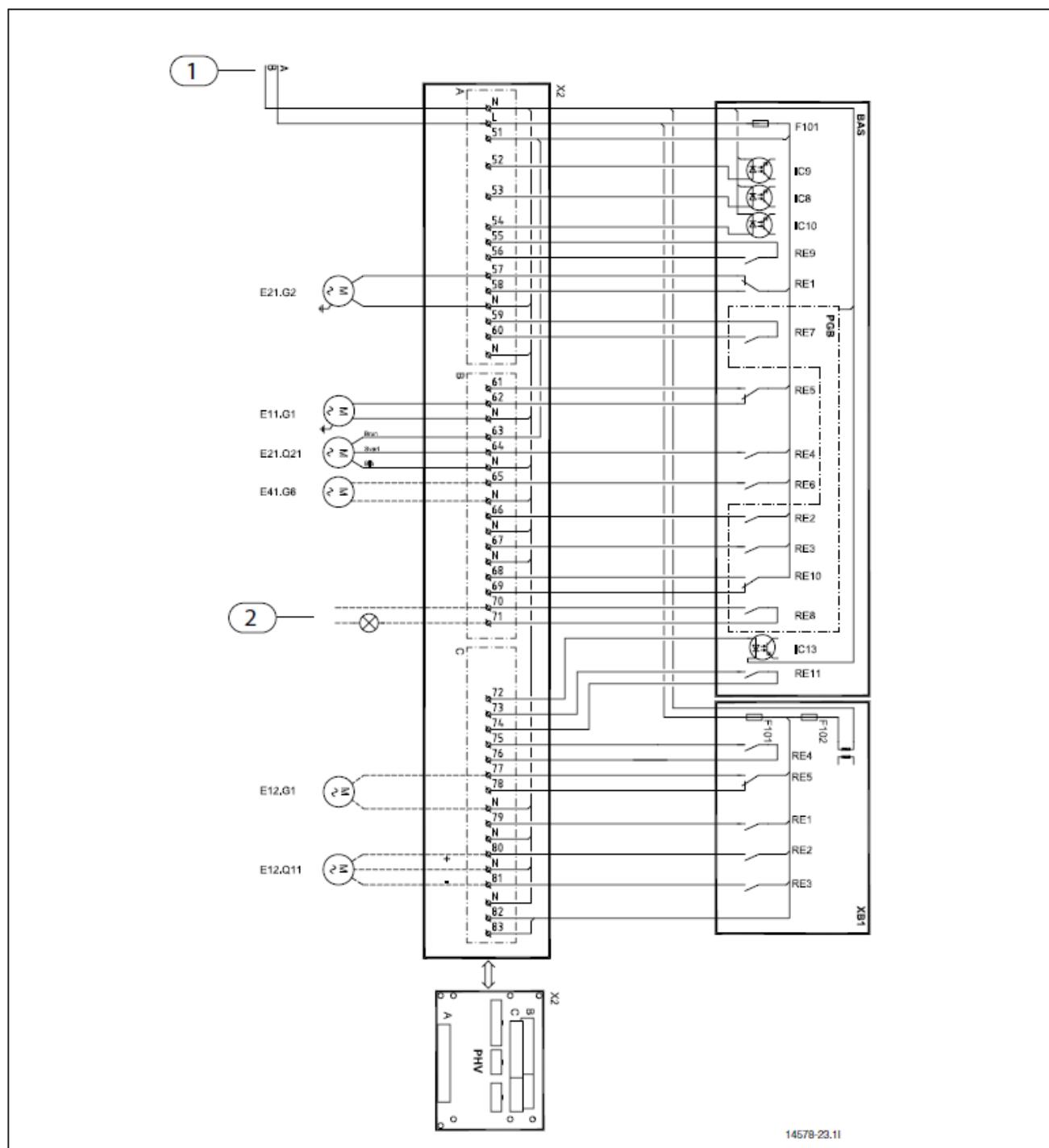
Bild 37 Anslutningar kombimodul
