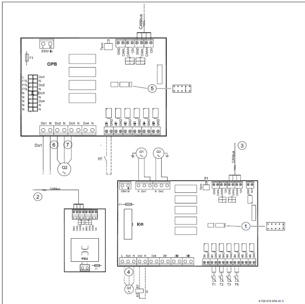
Bild 63 Externa anslutningar styrsåp, shuntat tillskott
