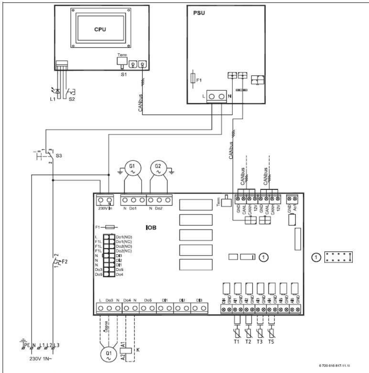
Bild 57 Kretsschema styrskåp
